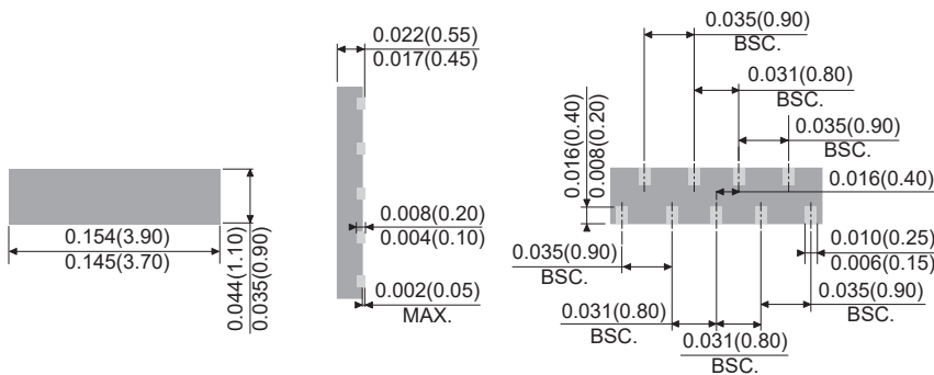
DFN3810-9L
