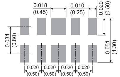
DFN3810-9L
